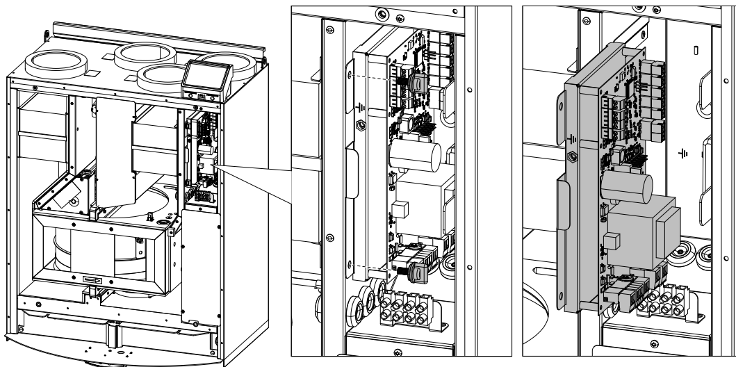
Рис. 4 Положение основной платы управления
