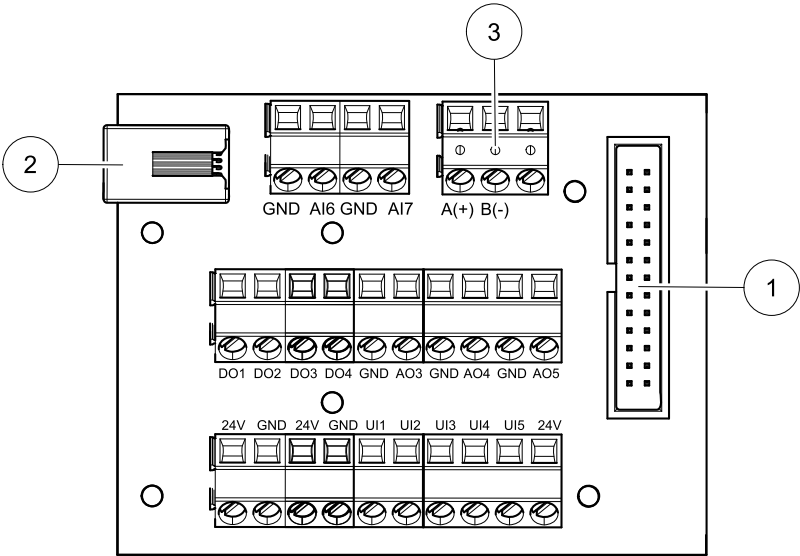
Рис. 6 Внешняя соединительная коробка и плата
