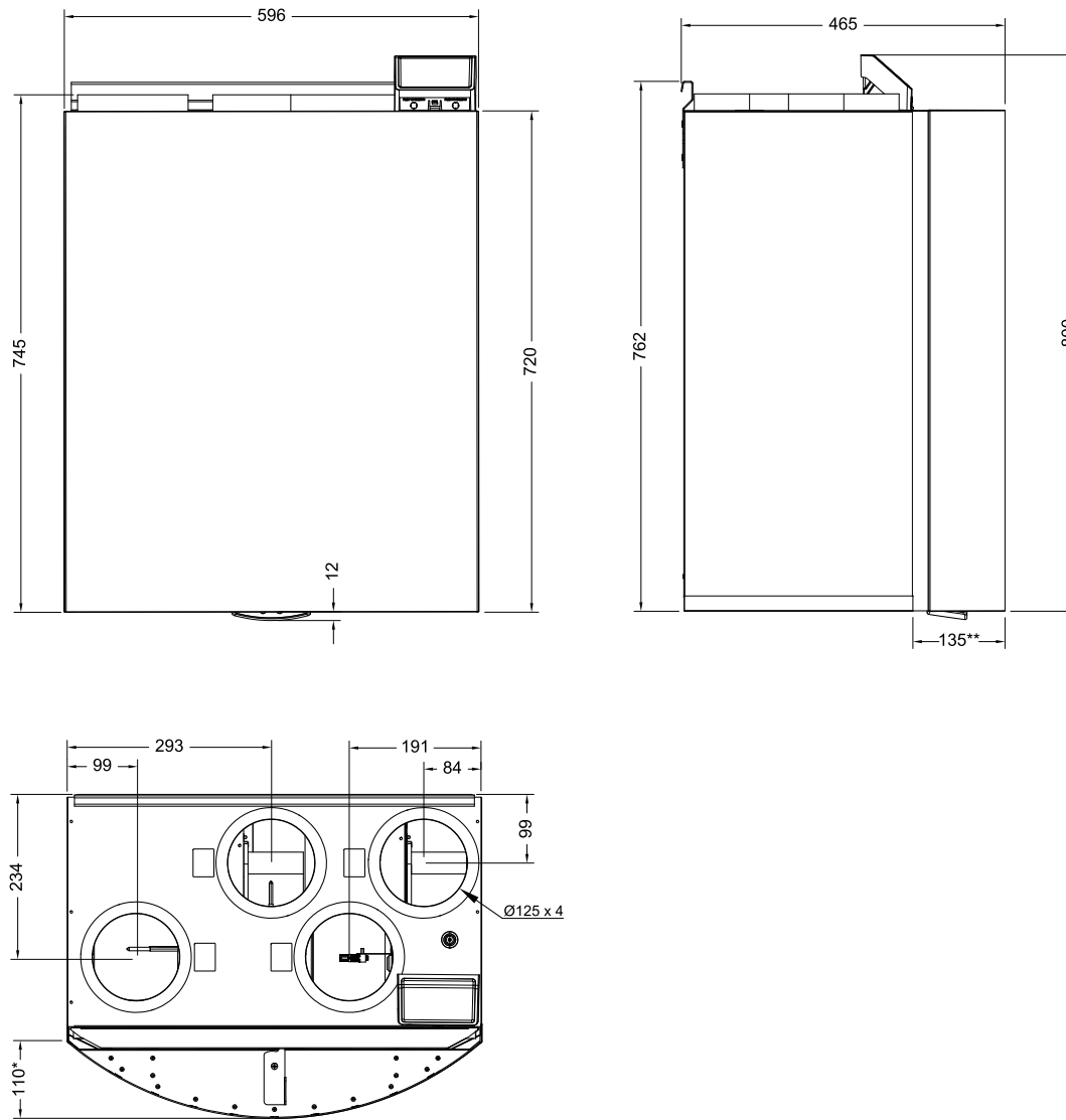
Рис. 2 Размеры и вес левосторонней модели (L)
